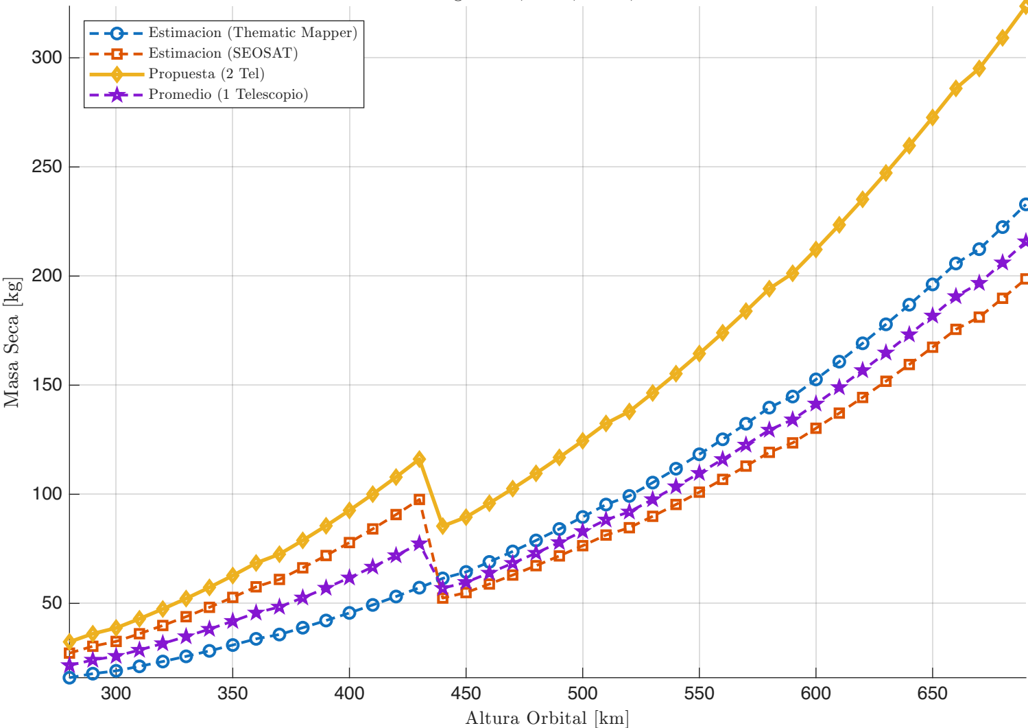
Comparativa de Masa Seca vs. Altura Config: 2 Sat, 2 Tel, Det 3, TMA
